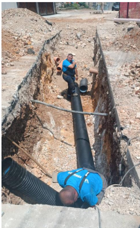
Slika br.14. Radovi na izgradnji atmosferske kanalizacije u dijelu ulice dr Slobodana Dragaševića (od raskrsnice sa ulicom Jadranska do raskrsnice sa Šavničkom ulicom)
