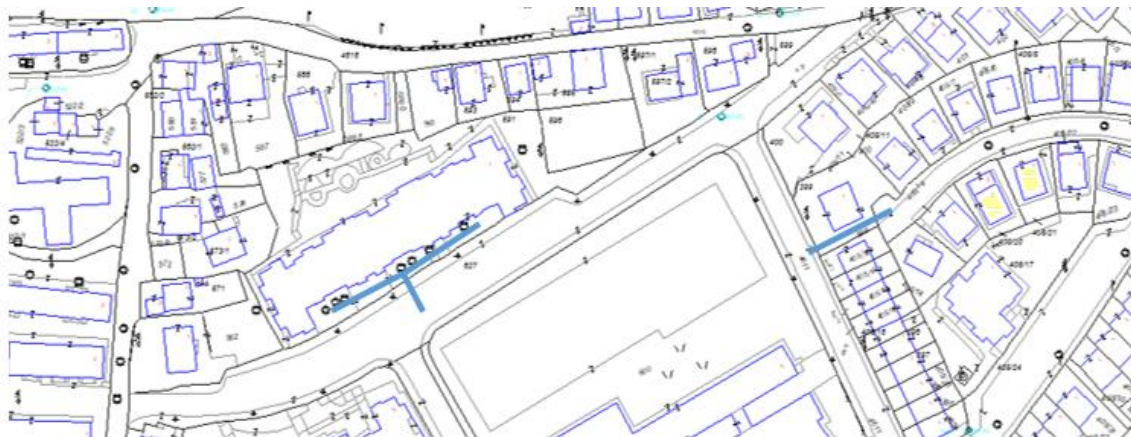
Slika br.1. Nastavak radova iz prethodne godine u ulicama Vlatka Samardžića i Baja Mirkovića
