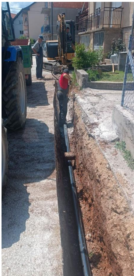
Slika br.4. Radovi na izgradnji vodovodne mreže u ulici dr Slobodana Dragaševića (od raskrsnice sa ulicom Save Kovačevića do raskrsnice sa Šavničkom ulicom)
